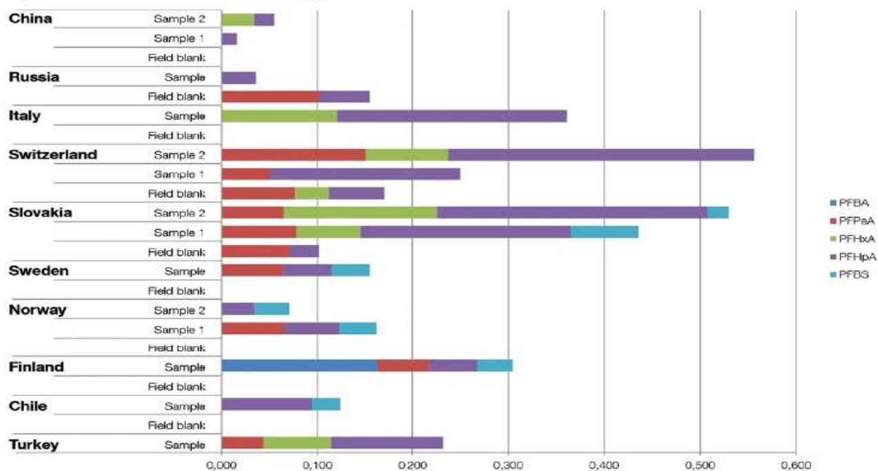
Figura 4. PFCs della catena corta nella neve, ng/l. (13)
