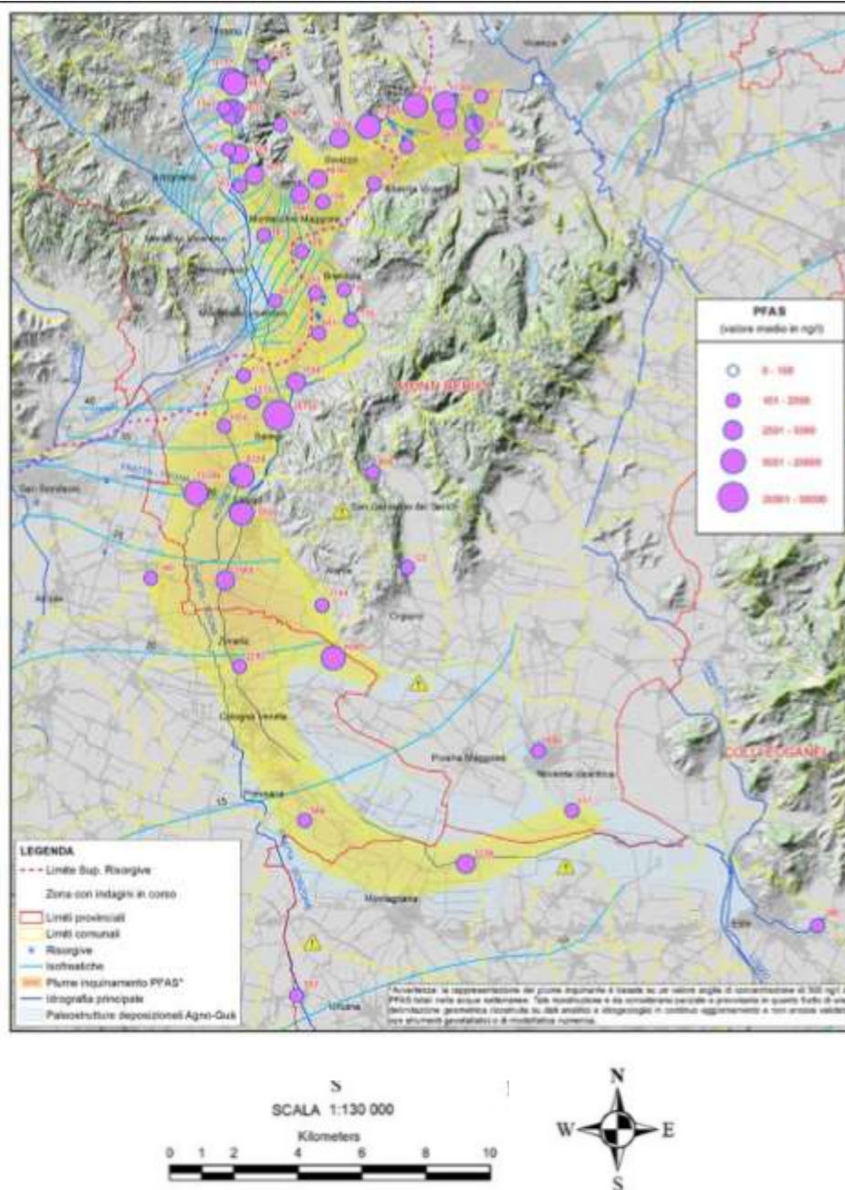
Figura 13. Monitoraggio dei PFAS nella rete di sorveglianza delle acque sotterranee, 2015-2016. Linea azzurra – isofreatica, linea blu – idrografia, linea gialla – limiti comunali, cerchi viola – concentrazione PFAS, ng/l; numeri in rosso – valore PFAS, ng/l (25)
