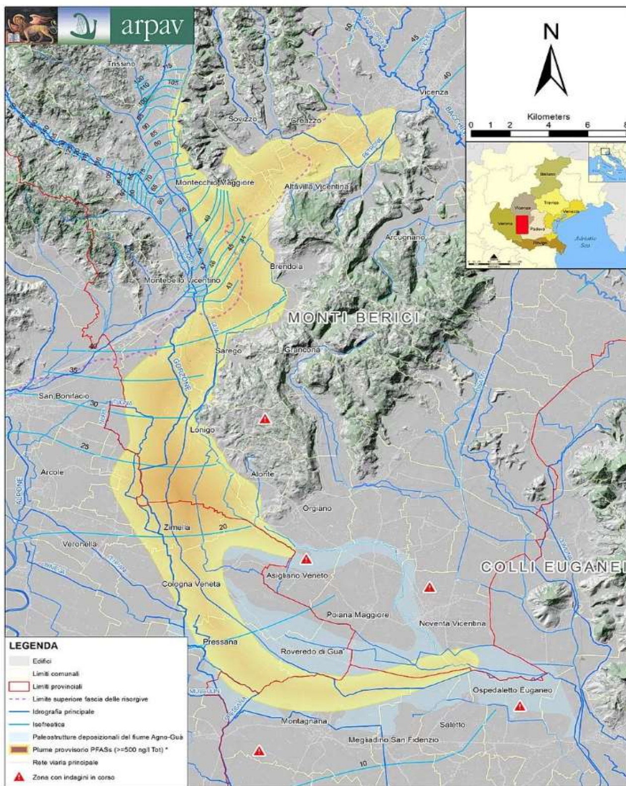
Figura 12. L'inquinamento da PFAS nelle province tra Vicenza, Verona e Padova, regione Veneto. Linea blu – idrografia, linea azzurra – isofreatica, punti rossi – zona di indagini in corso; colore giallo – plume provvisorio di inquinamento da PFAS di circa 40 km ( \geq 500 ng/l tot.) (36)
