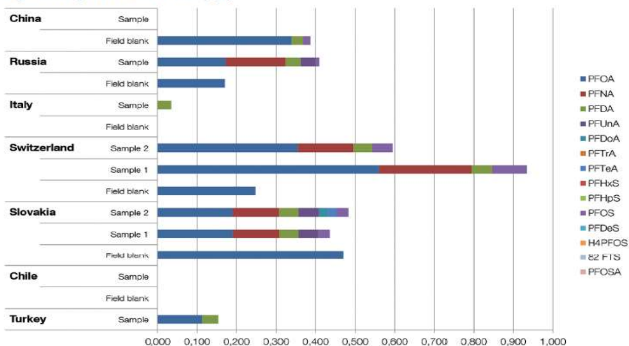
Figura 5. PFCs della catena lunga nell'acqua, ng/l. (13)
