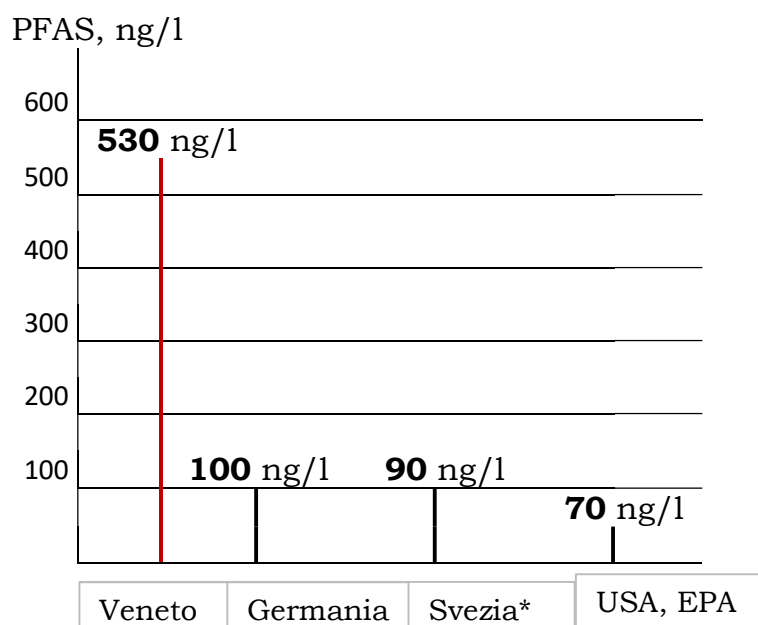
Figura 15. Confronto tra i livelli di sicurezza relativi alla presenza di alcuni PFAS (ng/l) nelle acque potabili.
