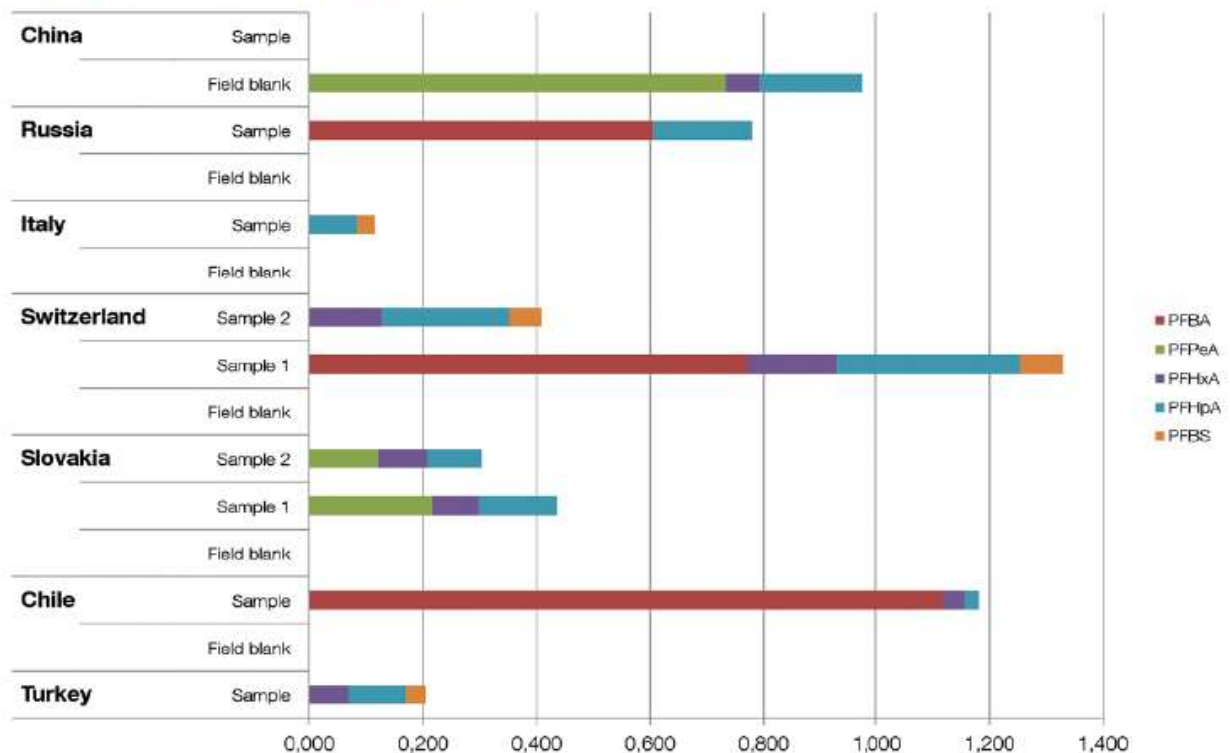
Figura 6. PFCs della catena corta nell'acqua, ng/l. (13)
