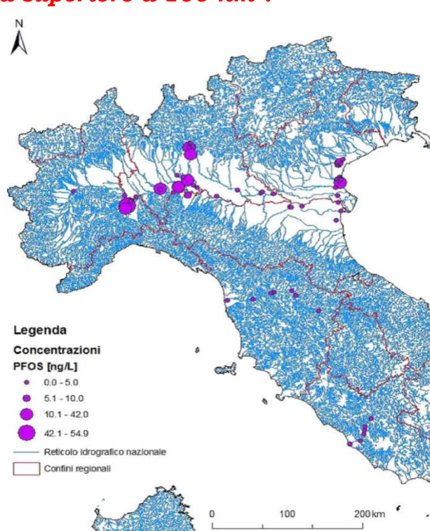
Figura 14. Le concentrazioni di PFOS (ng/l) in Italia. (36)
