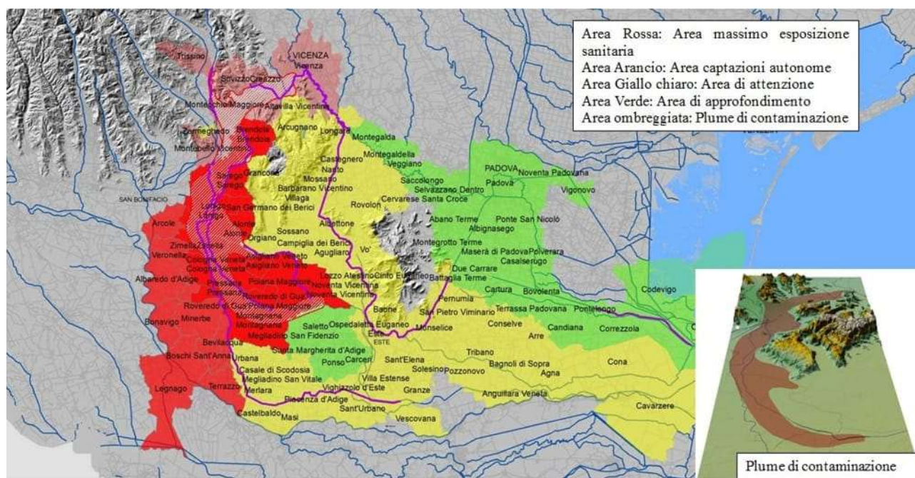
Figura 11. L'inquinamento da PFAS nelle province tra Vicenza, Verona e Padova, regione Veneto. Rosso: area massima esposizione sanitaria; arancio: area captazioni autonome; giallo: area di attenzione; verde: area di approfondimento; disegno a destra – plume di inquinamento. Provvisorio. (14, rapporto della Commissione Parlamentare, 08.02.2017)
