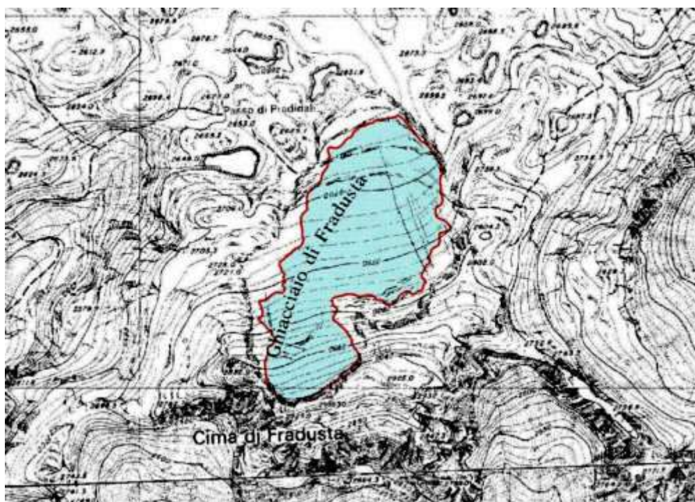
Fig. 9. Il ghiacciaio Fradusta (2)
