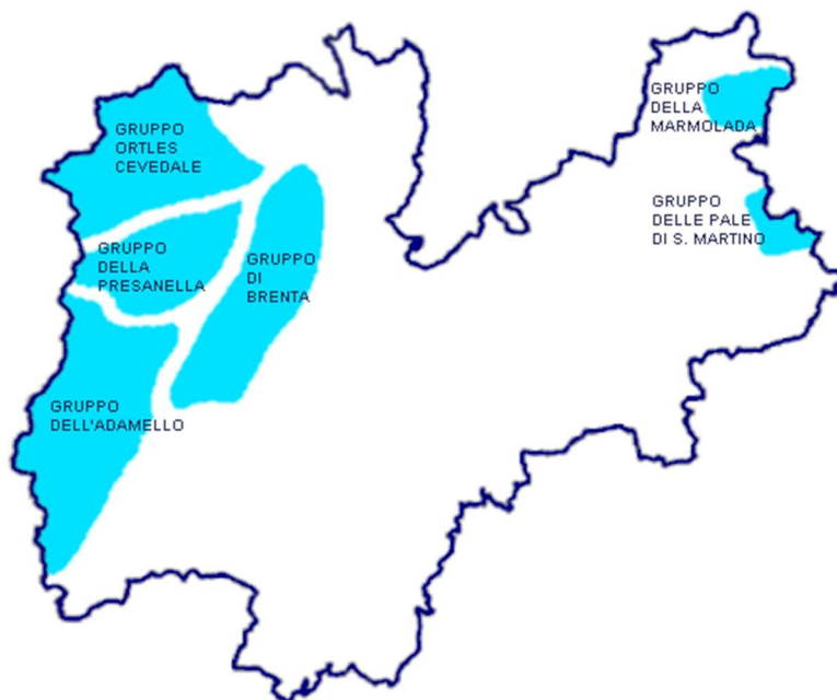
Fig. 4. Suddivisione dei Ghiacciai secondo la Società degli Alpinisti Tridentini (2)
