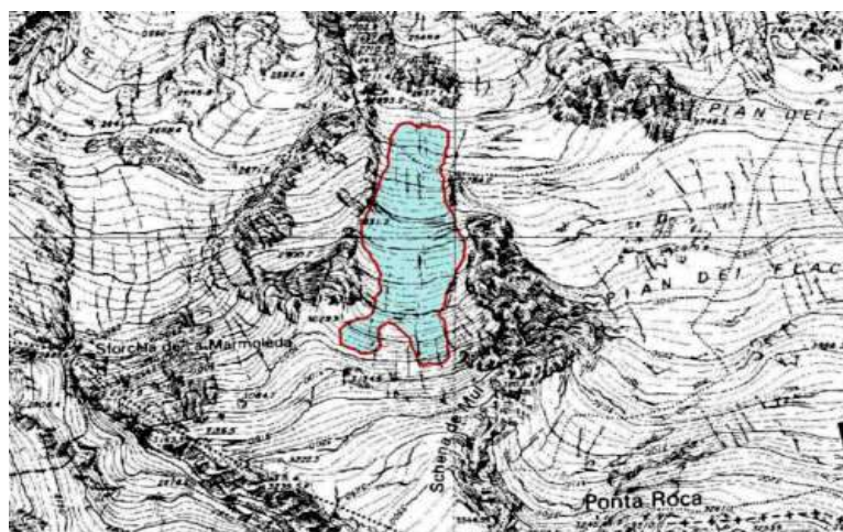
Fig. 6. Il ghiacciaio Occidentale del Vernel (Gruppo Marmolada). (2)
