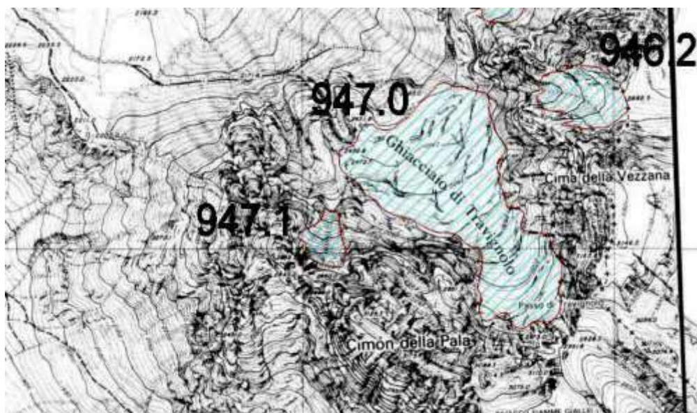
Fig. 10. Il ghiacciaio di Travignolo
