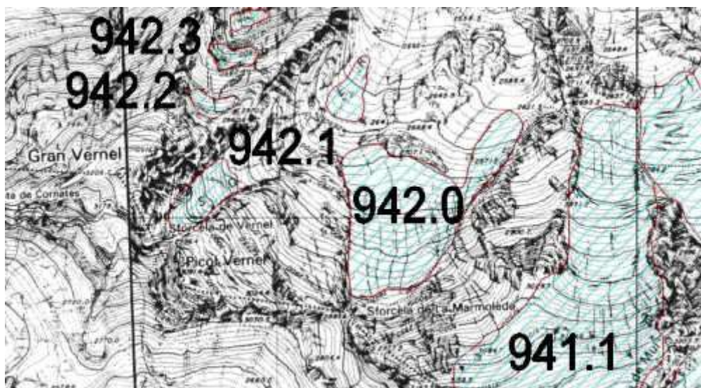
Fig. 7. Il ghiacciaio Occidentale della Marmolada (2)
