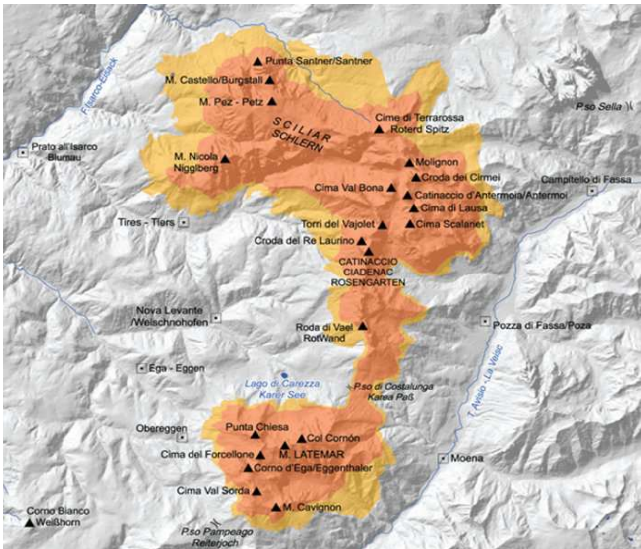
Fig. 3. Sistema 7 – Sciliar-Catinaccio, Latemar
