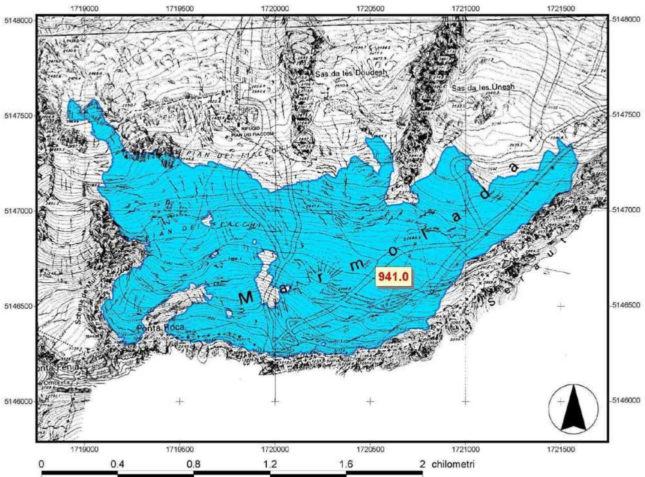
Fig. 5. La superficie del Ghiacciaio Principale della Marmolada nel 1994 (2)
