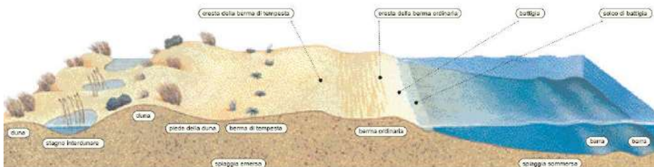
Figura 10. Profilo dunale costiero.
