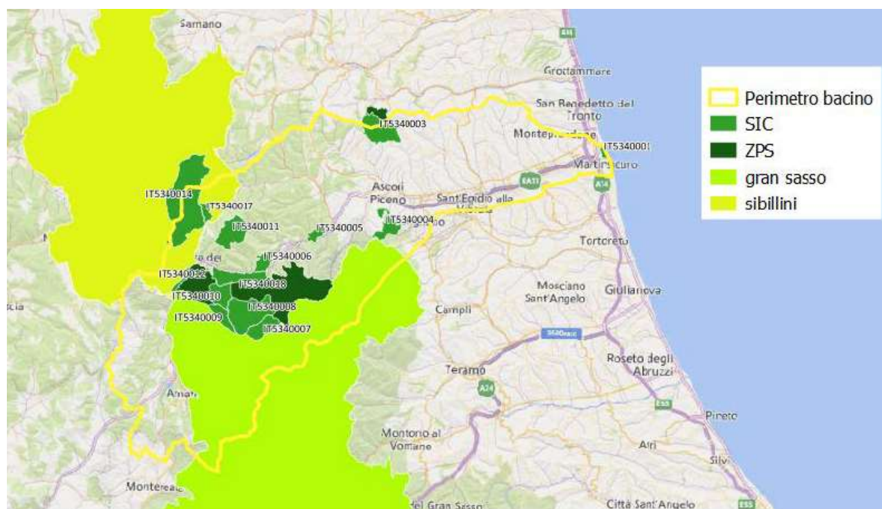
Figura 14. Parchi Nazionali, le aree SIC e ZPS nel bacino del fiume Tronto. (7)
