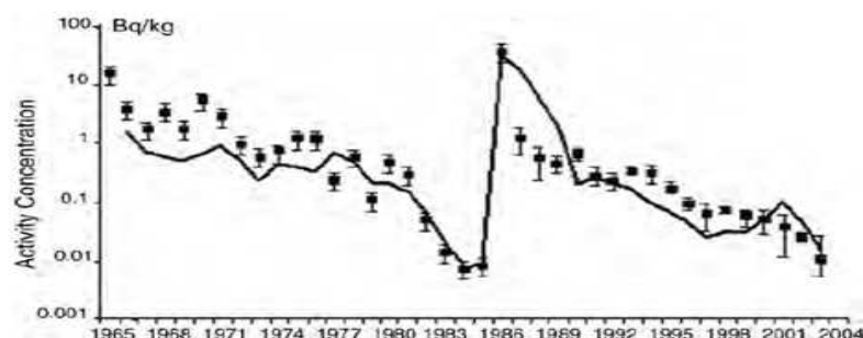
Fig.53. La concentrazione del Cs-137 nel frumento (Bq/kg) in Croazia dal 1965 al 2004 (Franic et al., 2006).
