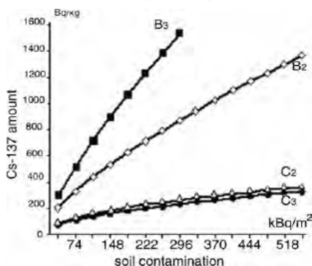
Fig. 27. Contenuto del Cs-137 (Bq/kg) nei mirtilli Vaccinum myrtillus e nel suolo, KBq/m 2 , in Ucraina).
