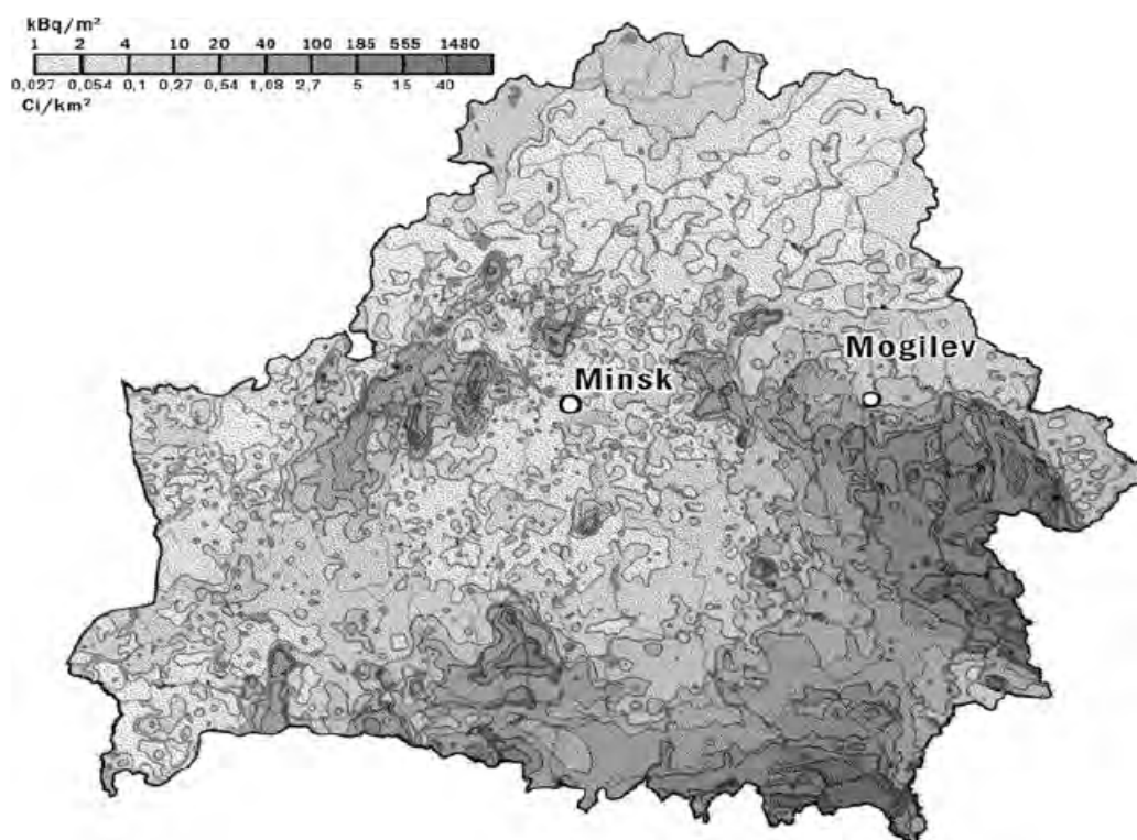
Fig.4. Ricostruzione della contaminazione da Cs-137 in Bielorussia, 10.05.1986 (National Belarussian Report, 2006).
