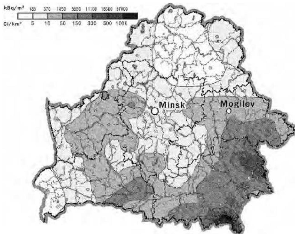
Fig.2. Ricostruzione della contaminazione da I-131 in Bielorussia, 10.05.1986 (National Belarussian Report, 2006).
