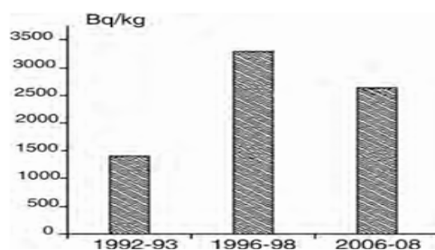
Fig. 36. La concentrazione media del Cs-137 (Bq/kg del peso umido) nei muscoli di alce ( Alces alces ) sul suolo contaminato della provincia di Bryansk, Russia (Pel'gunov et al., 2006)
