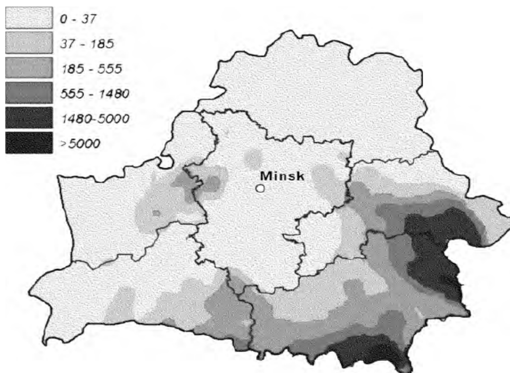
Fig.3. Ricostruzione della contaminazione da Te-132 e I-131 in Bielorussia, aprile-maggio 1986 (Zhuravkov and Mironov, 2005).
