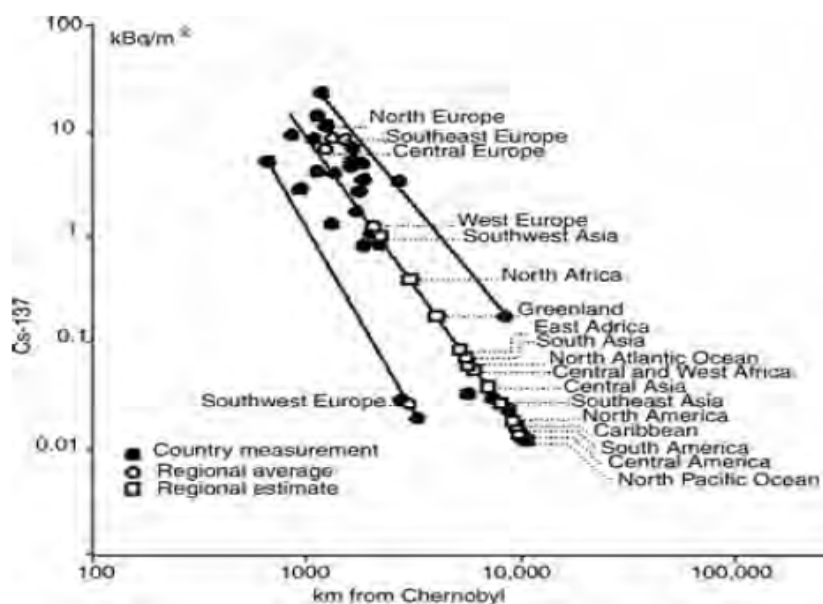
Fig. 1. La distribuzione geografica dei radionuclidi di Chernobyl (UNSCEAR, 1988)
