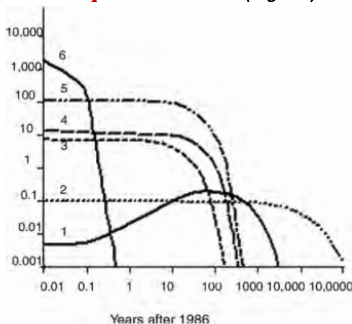
Fig.59. Radioattività totale aggiuntiva (in petabecquerel, PBq ( 10^{15} )) all'ambiente globale dopo la catastrofe Di Chernobyl: 1 – Am-241, 2 – Pu (239+240), 3 – Pu-241, 4 – Sr-90, 5 – Cs-137, 6 – I-131 (Mulev, 2008)
