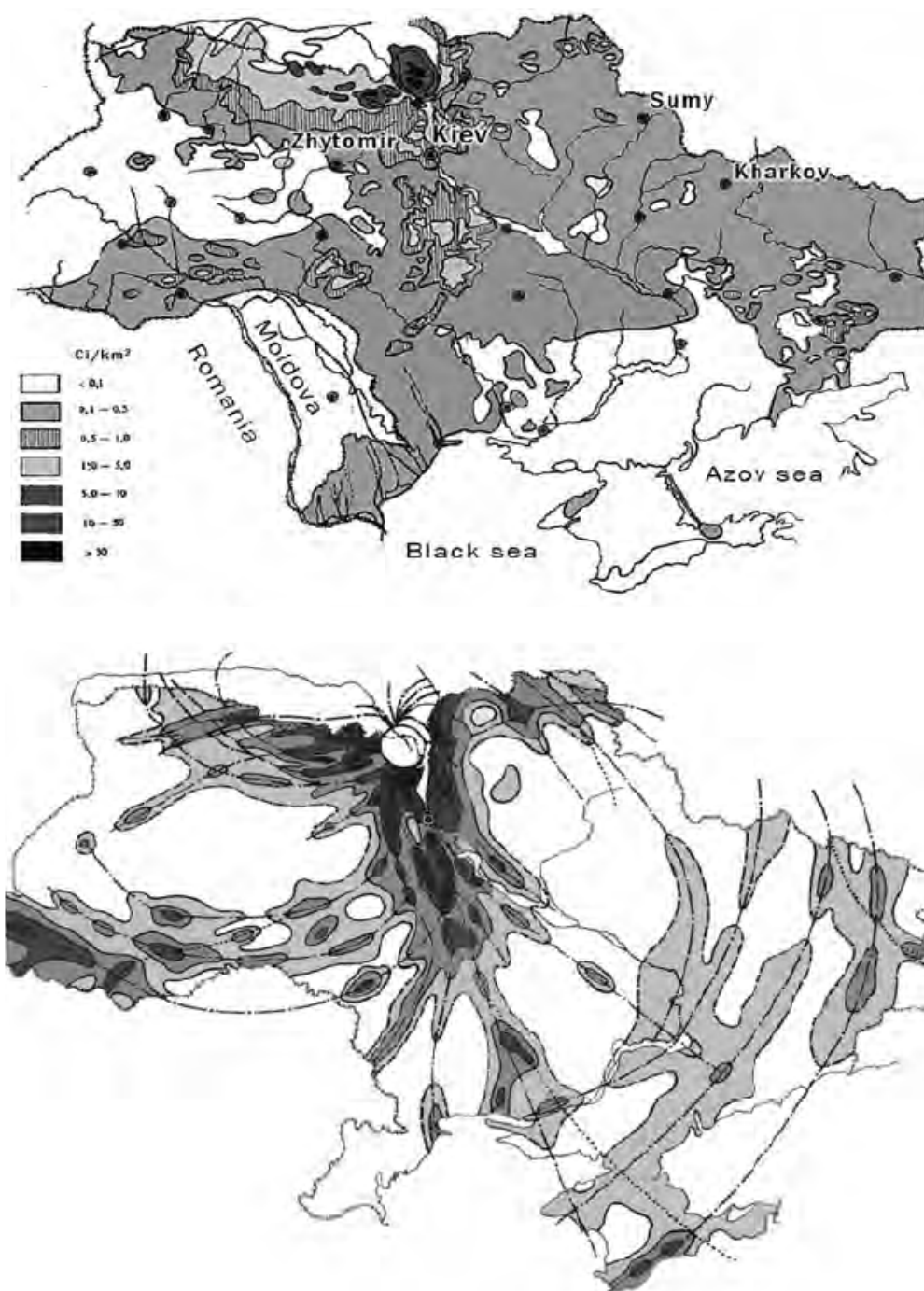
Fig.5. La contaminazione del territorio dell'Ucraina da Cs-137 (sopra) e da Plutonio (Pu) (sotto) dopo la catastrofe sulla centrale nucleare di Chernobyl (National Report of Ucraina, 2006).
