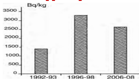
Рис. 36. Средняя концентрация цезия Cs-137 (Бк/кг, сырой вес) в мышцах лося ( Alces alces ) на загрязненной территории Брянской области, Россия (Pel'ginov et all., 2006)
