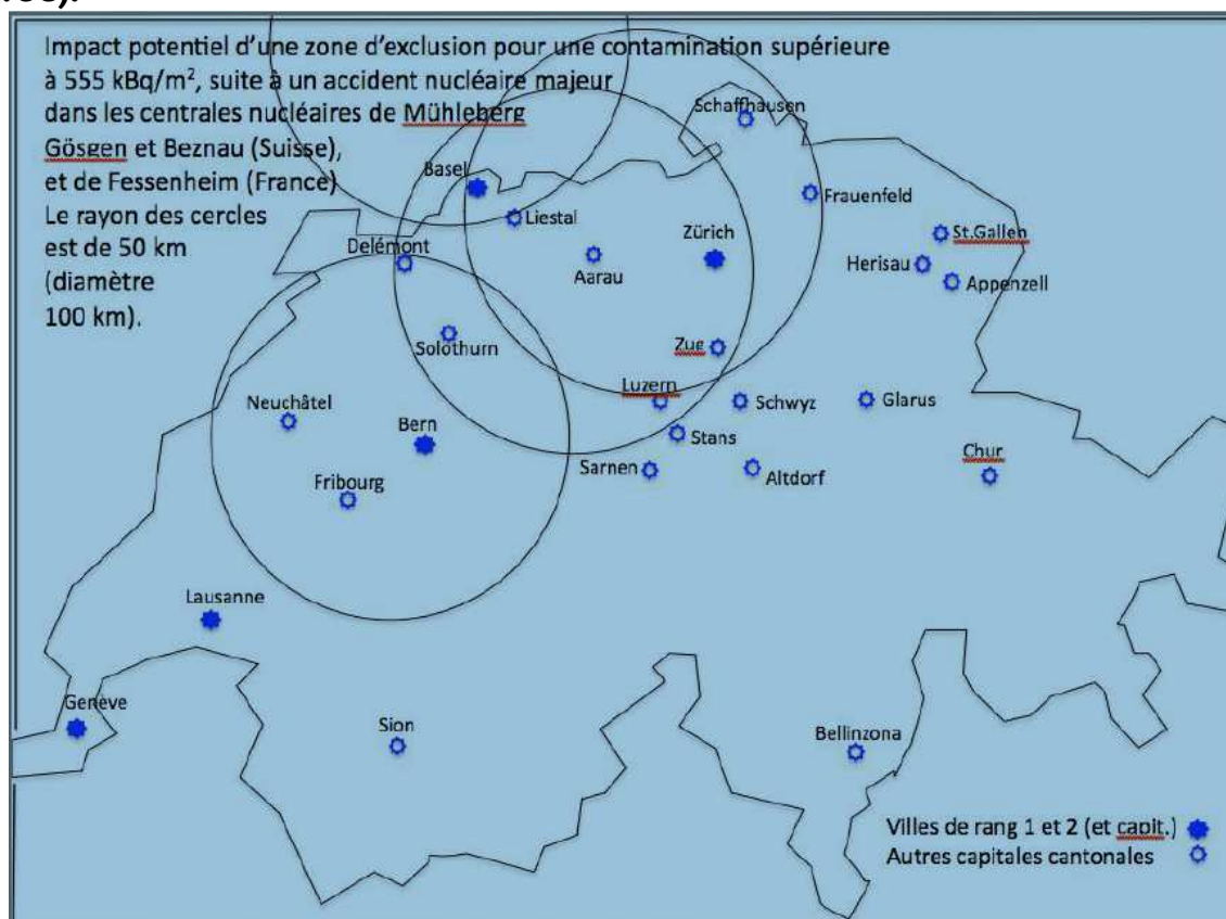
Рис.63. Потенциальный эффект в случае загрязнения более 555 КБк/м 2 (зона отселения – радиус 50 км) в случае серьезной атомной аварии на АЭС в г.Мюхлеберг (круг слева), АЭС Безнау (круг справа), АЭС Госген (Швейцария) (круг в центре) и в г.Фессенхейм (Франция) (круг сверху). (8)
