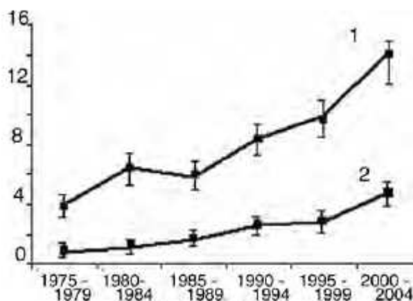
Рис. 12. Частота заболеваемости раком щитовидной железы (на 100'000 человек) в провинции Марн-Арденн, Франция, 1975-2004 г.г. (Cherie-Challine et al., 2006).
