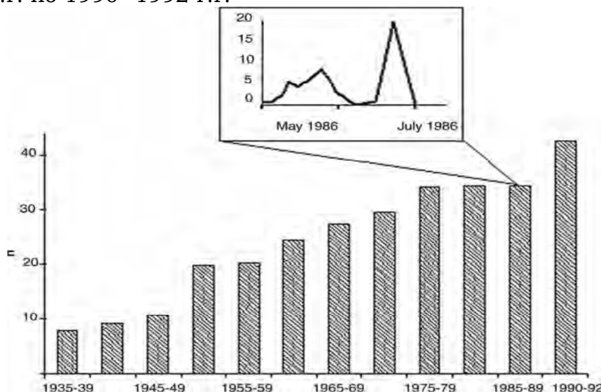
Рис. 15. Частота заболеваемости раком щитовидной железы среди детей (на 1'000'000 ) с 1935 по 1992 г.г. и концентрация йода I-131 в молоке в штате Коннектикут (Reid and Mangano, 1995)
