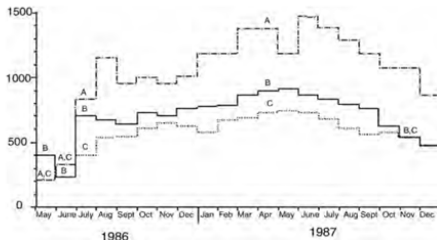
Рис.56. Нагрузка организма за счет цезия Cs-137 (Бк) в организме человека в г.Мюнхен, Германия, и в г.Гренобль, Франция, 1986-1987: (А) мужчины, (В) женщины, (С) взрослые в Гренобле, Франция (В) (UNSCEAR, 1988).
