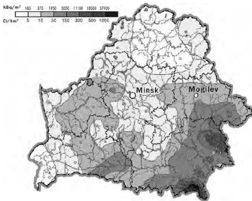
Рис.2. Реконструкция загрязнения йодом I-131 в Белоруссии, 10.05.1986 г. (Белорусский Национальный Отчет, 2006 г.).
