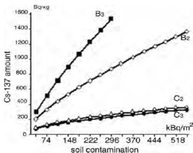
Рис. 27. Содержание цезия Cs-137 (Бк/кг) в ягодах черники Vaccinium myrtillus и в почве, КБк/м 2 , Украина.
