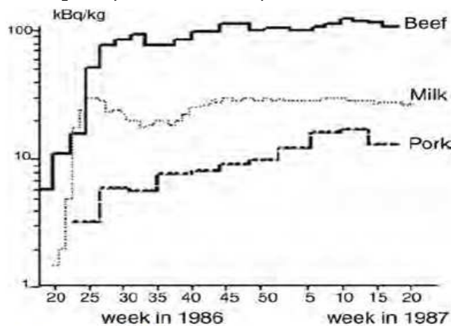
Рис.50. Концентрация цезия Cs-137 в мясе и молоке в Финляндии, КБк/кг. (UNSCEAR, 1988, свержу – говядина, молоко, мясо свинина).
