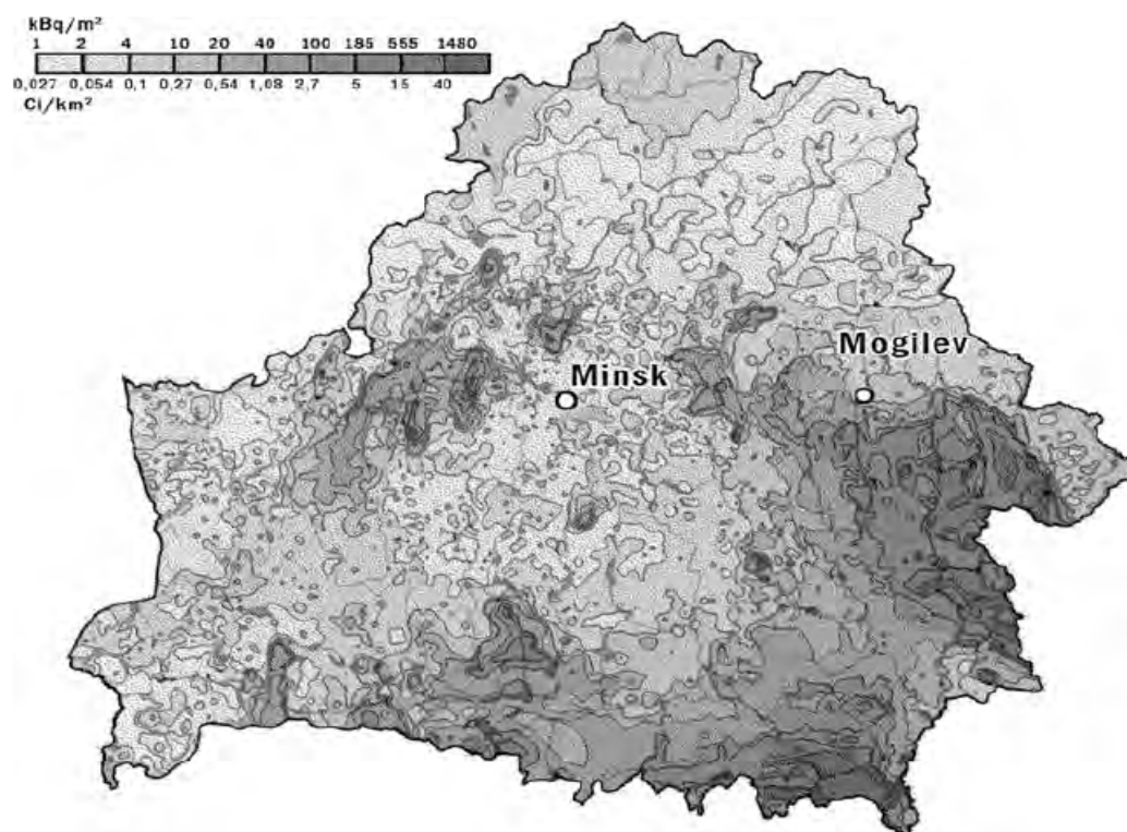
Рис.4. Реконструкция загрязнения цезием \text{Cs-137} в Белоруссии, 10.05.1986 г. (Белорусский Национальный Отчет, 2006 г.).
