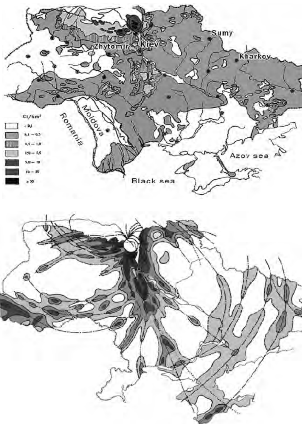
Рис.5. Загрязнение территории Украины цезием Cs-137 (сверху) и плутонием (Pu) (внизу) после аварии на Чернобыльской атомной станции (Национальный Отчет Украины, 2006 г.).
