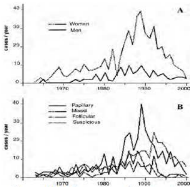
Рис. 13. Частота встречаемости гистологически различных типов рака щитовидной железы среди женщин (А, линия сверху) и среди мужчин (А, линия внизу) в Греции в 1963-2000 г.г. (Plias et all., 2002)
