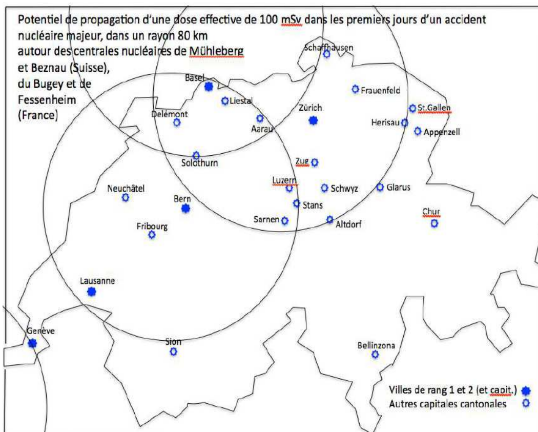
Рис.62. Потенциальное распространение эффективной дозы в 100 мЗв в первые дни серьезной атомной аварии в радиусе 80 км вокруг АЭС г. Мухлеберг (круг слева), г.Безнау (круг справа), г.Бугей (Швейцария) и г.Фессенхейм (Франция) (круг сверху). (8)
