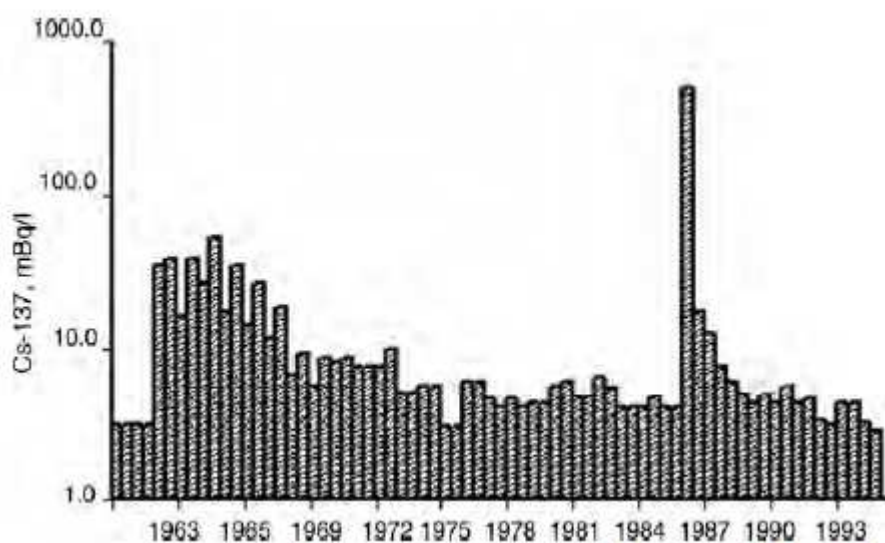
Рис.24. Концентрация Cs-137 (мБк/л) в поверхностных водах Тирренского моря, 1960-1995 г.г. (Europe Environmental Agency, 1999).
