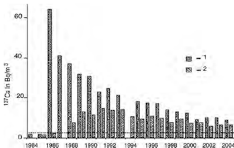
Рис. 52. Средняя годовая концентрация цезия Cs-137 (Бк/кг) в мускулах речной камбалы ( Platichthys flesus ) и морской камбалы ( Pleuronectes platessa ) с 1984 по 2004 с острова Bornholm и Балтийского моря, южная часть. Значение до-Чернобыль для обоих видов было 2,9 (HELCOM Indicator Fact Sheets. 2006. Online 22.04.2008; // www.helcom.fi/environment2/ifs/en_GB/cover/ )
