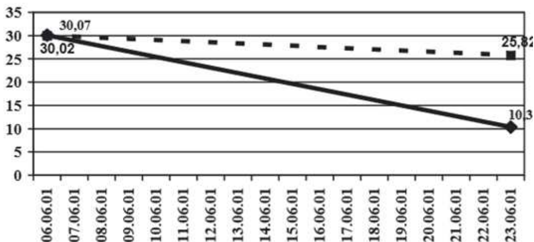
Рис.57. Уровень уменьшения удельной активности Cs-137, Бк/кг, после приема добавок Vitapect (линия внизу) и Placebo (линия сверху) с 06 по 23 июня 2001 г. (3)
