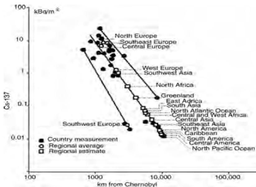
Рис. 1. Географическое распределение радионуклидов после Чернобыльской аварии (UNSCEAR, 1988)
