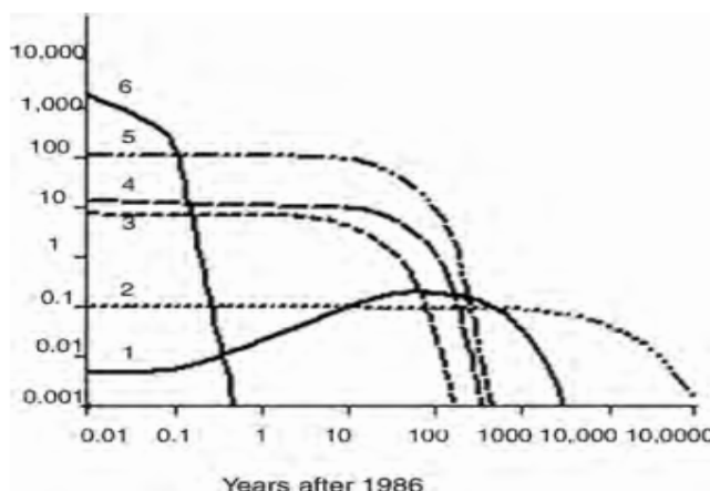
Рис.59. Общая дополнительная радиоактивность (в петабеккерелях, ПБк ( 10^{15} )) в глобальной окружающей среде после Чернобыльской аварии: 1 – Am-241, 2 – Pu (239+240), 3 – Pu-241, 4 – Sr-90, 5 – Cs-137, 6 – I-131 (Mulev, 2008)
