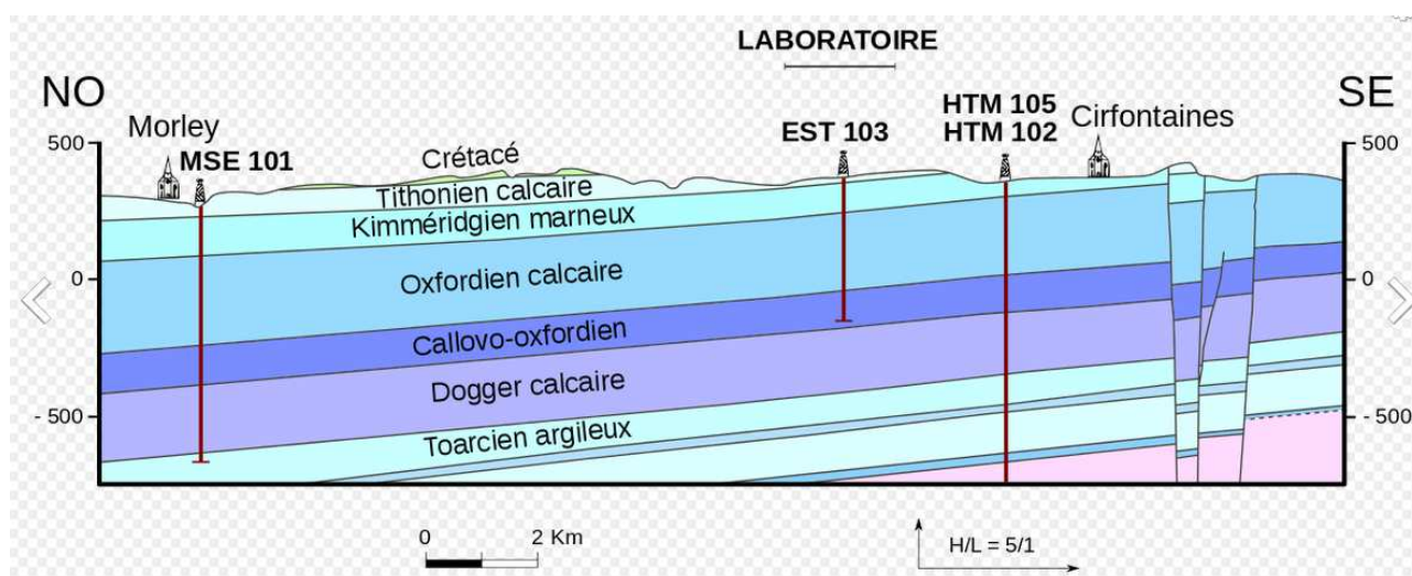
Figura 15. Profilo geologico del sito Bure.
