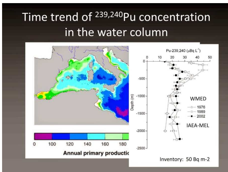
Figura 19. La concentrazione di plutonio - 239, 240 (μBq/l) in una colonna d'acqua a dipendenza di profondità (0 - -2'500 m) nel Mediterraneo.
