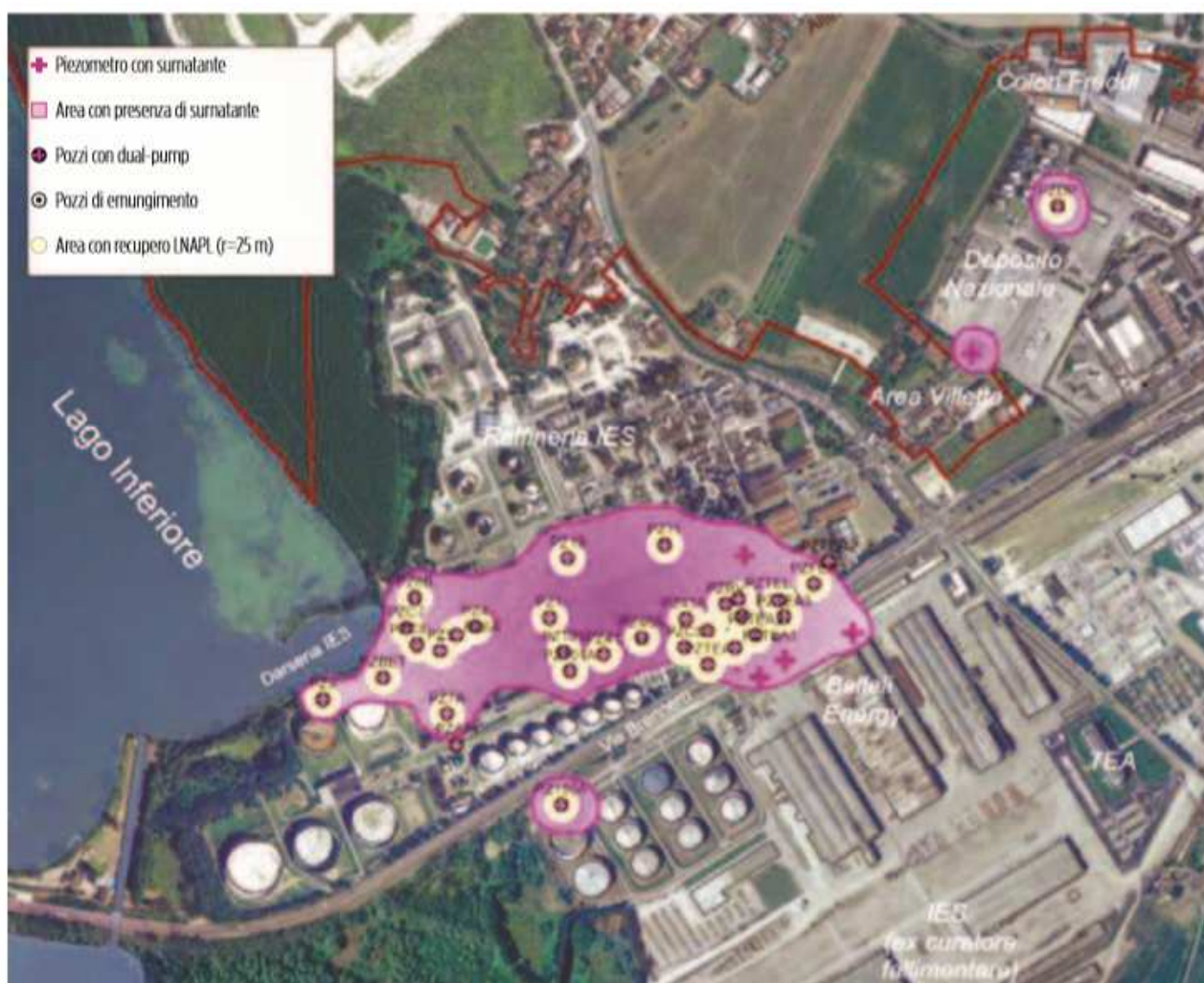
Figura 16. Distribuzione del urnatante presso la raffineria IES di Mantova, giugno, 2009. La crocetta rosa – piezometro con surnatante, colore rosa – area con presenza di surnatante (1)
