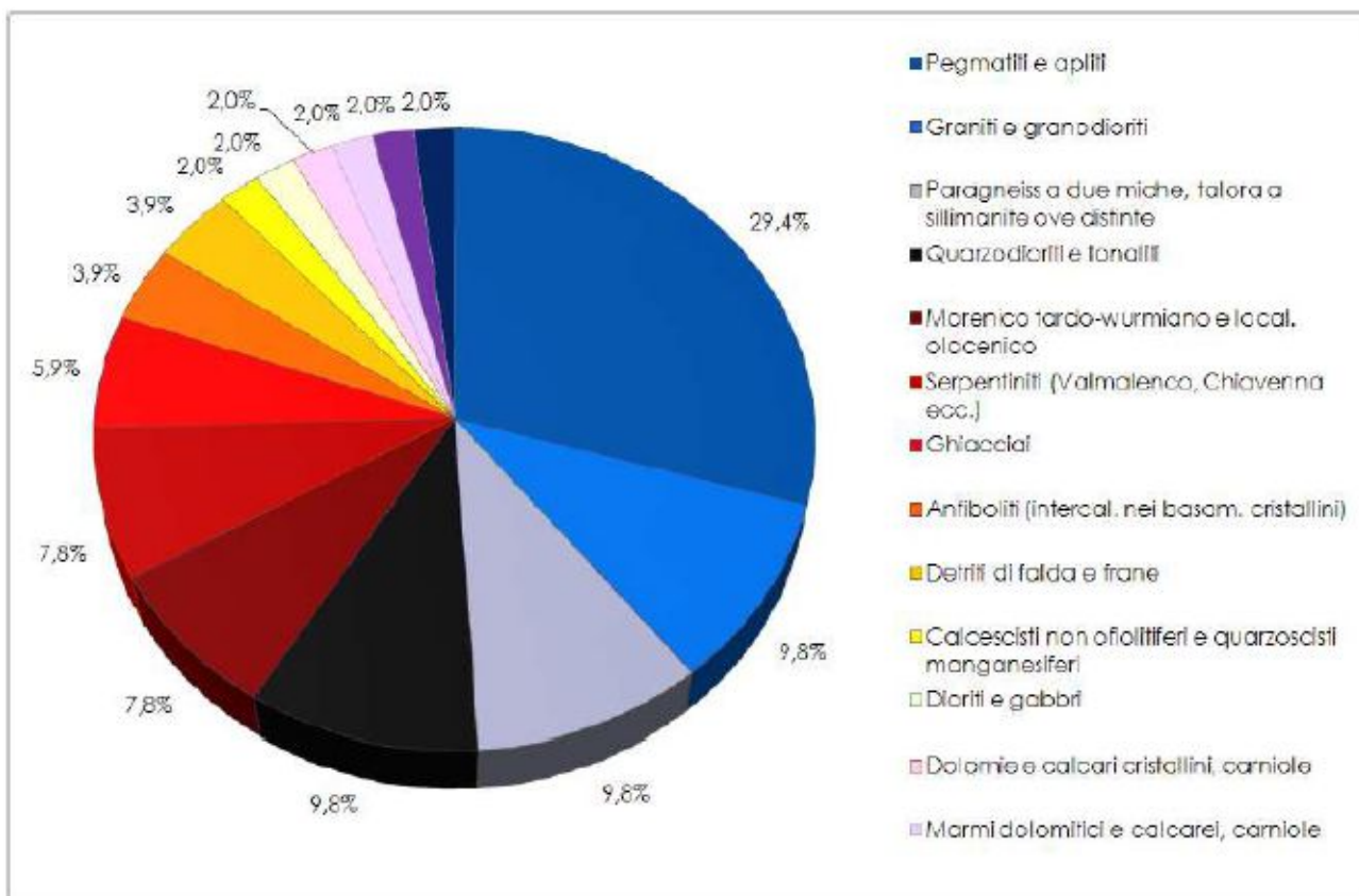
Рисунок 31. Состав геологического субстрата в зоне ZPS (%). (25)
